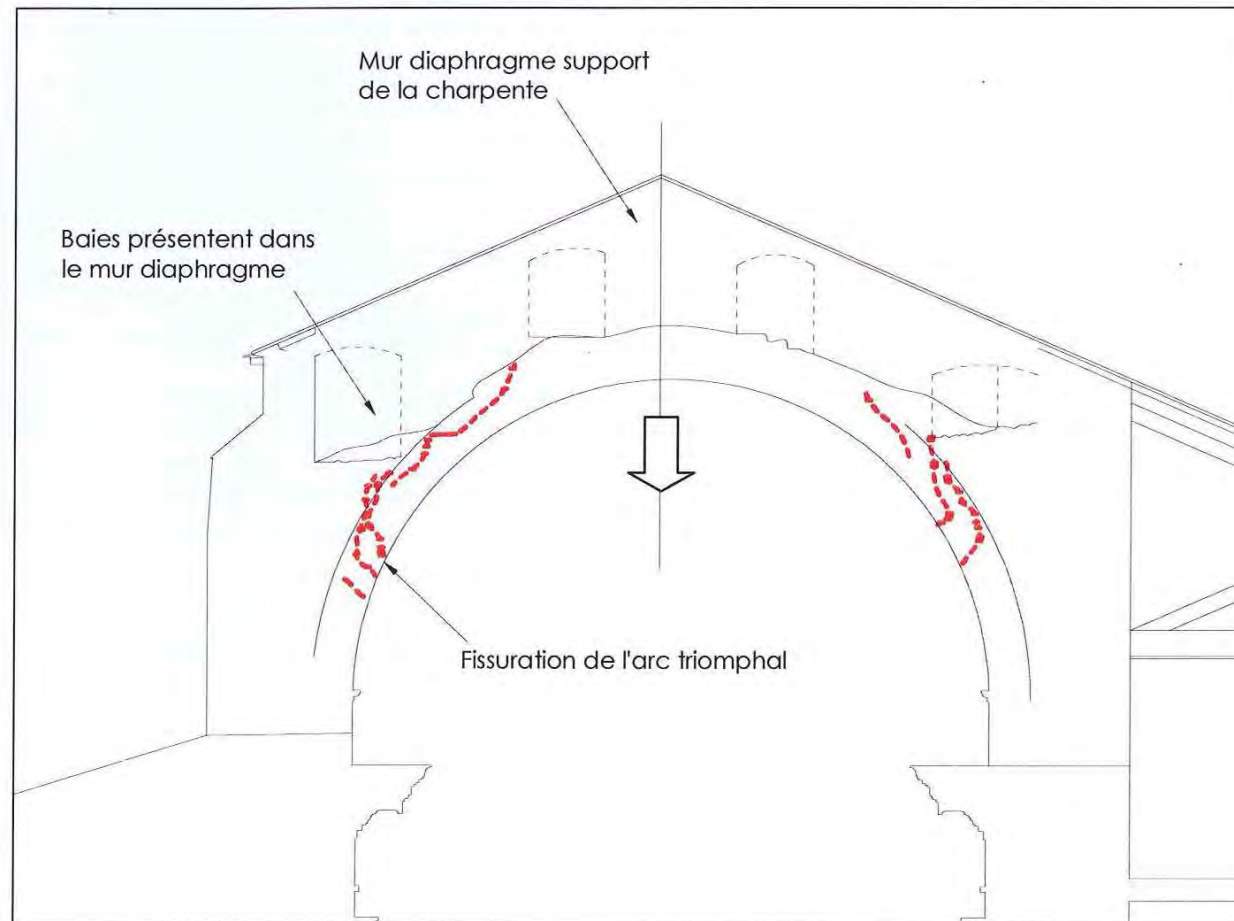
Figure 8 Coupe transversale sur arc triomphal - Définition des désordres
