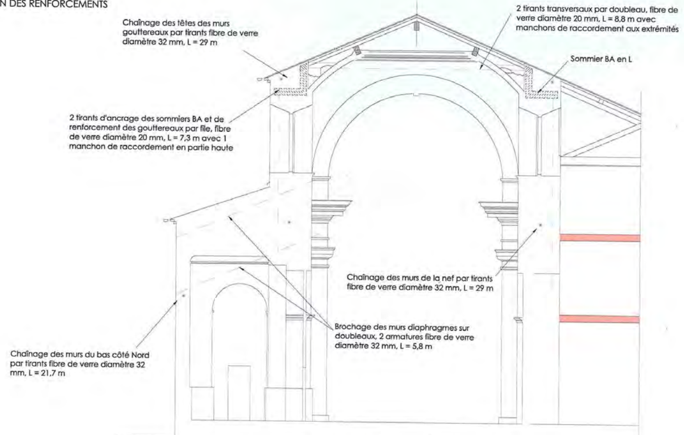
COUPE AA
